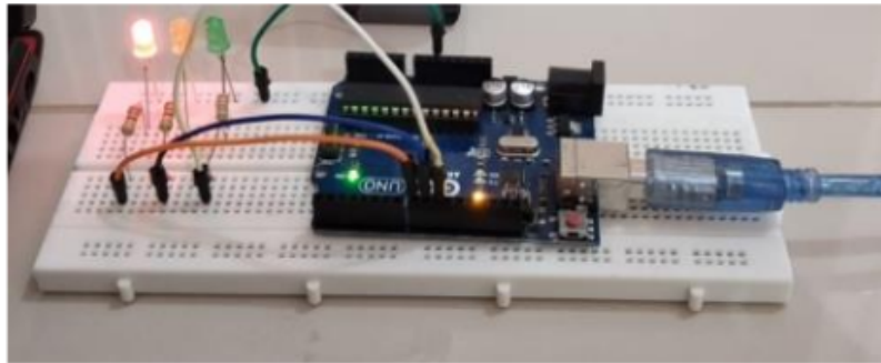
Gambar 4.49. Hasil Perakitan Rangkaian LED Indikator
