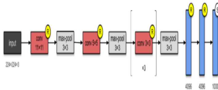
Gambar 1.2. Arsitektur Alexnet
