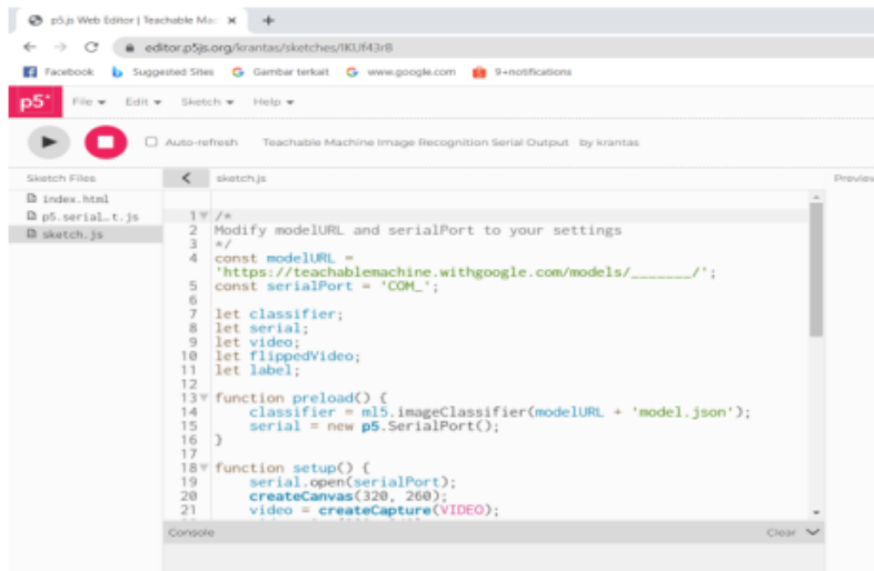
Gambar 4.54. Link Editor.p5js.org
