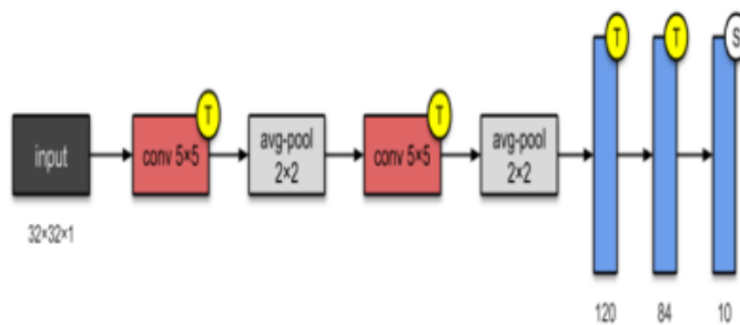
Gambar 1.1. Arsitektur Lenet
