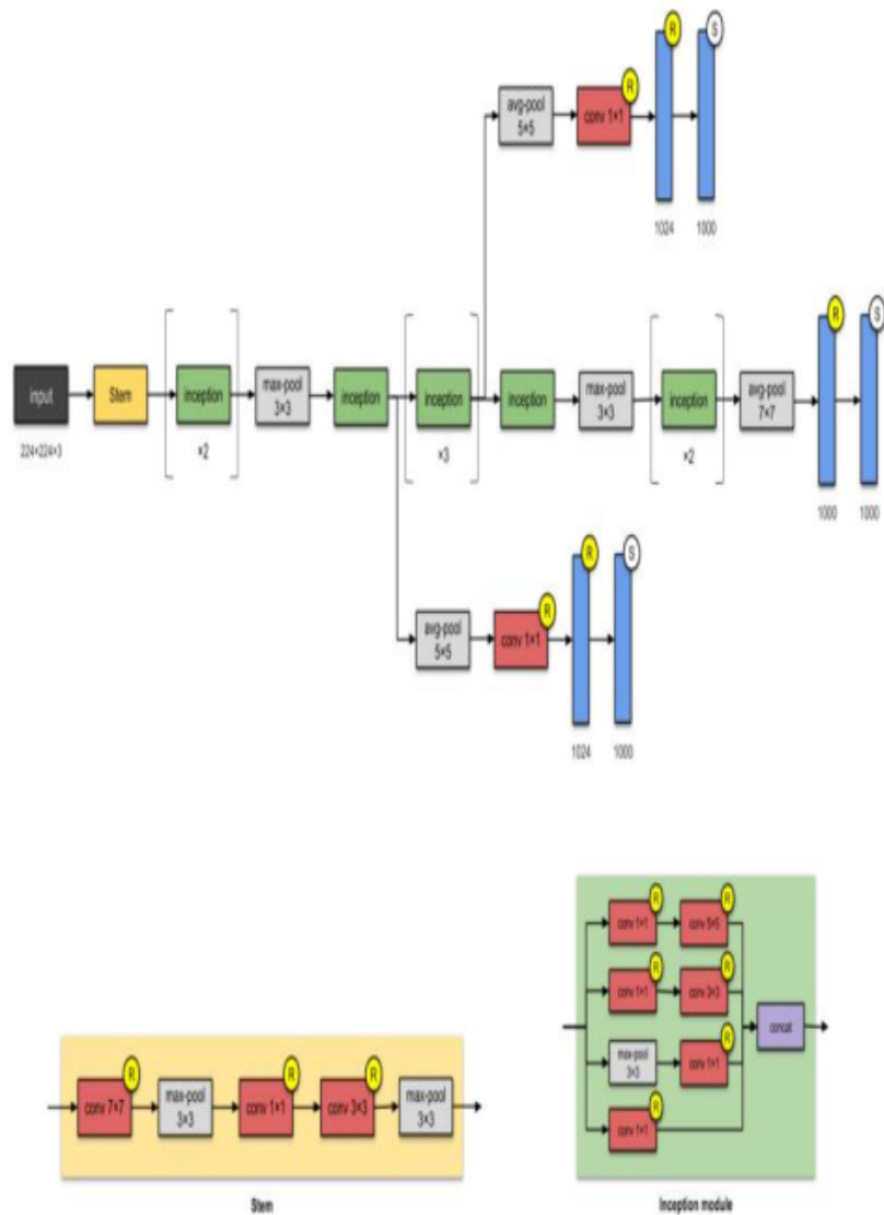
Gambar 1.4. Arsitektur Inception-v1
