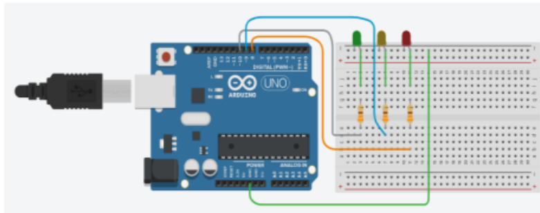
Gambar 4.41. Skema Rangkaian Arduino Uno R3 dengan 3 buah LED Indikator
