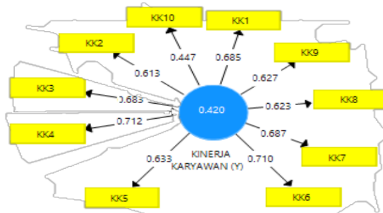
Gambar 2. Output Statistik
