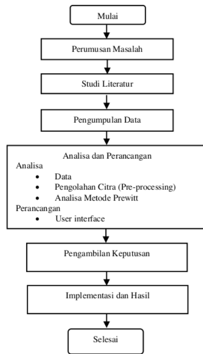
Gambar 1. Metodologi Penelitian
