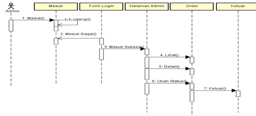
Gambar 1.12 Sequence Diagram Kelola Order oleh Admin
