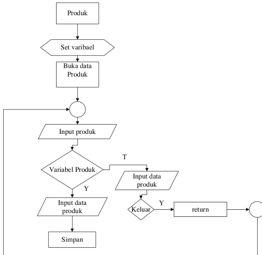
Gambar 1.32 Flowchart Input Produk
