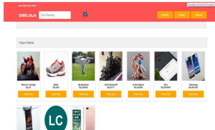
Gambar6.7 Antarmuka HalamanUtama
