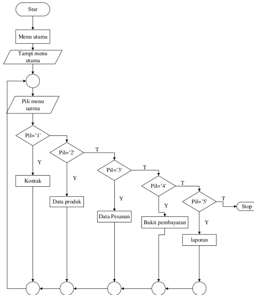
Gambar 1.31Flowchart Menu Utama
