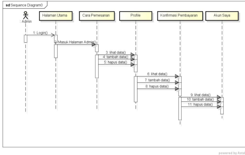
Gambar 1.10 Sequence Diagram Kelola Data Produk Admin
