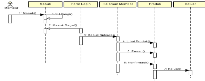
Gambar 1.11 Sequence Diagram Kustomer Melakukan Order
