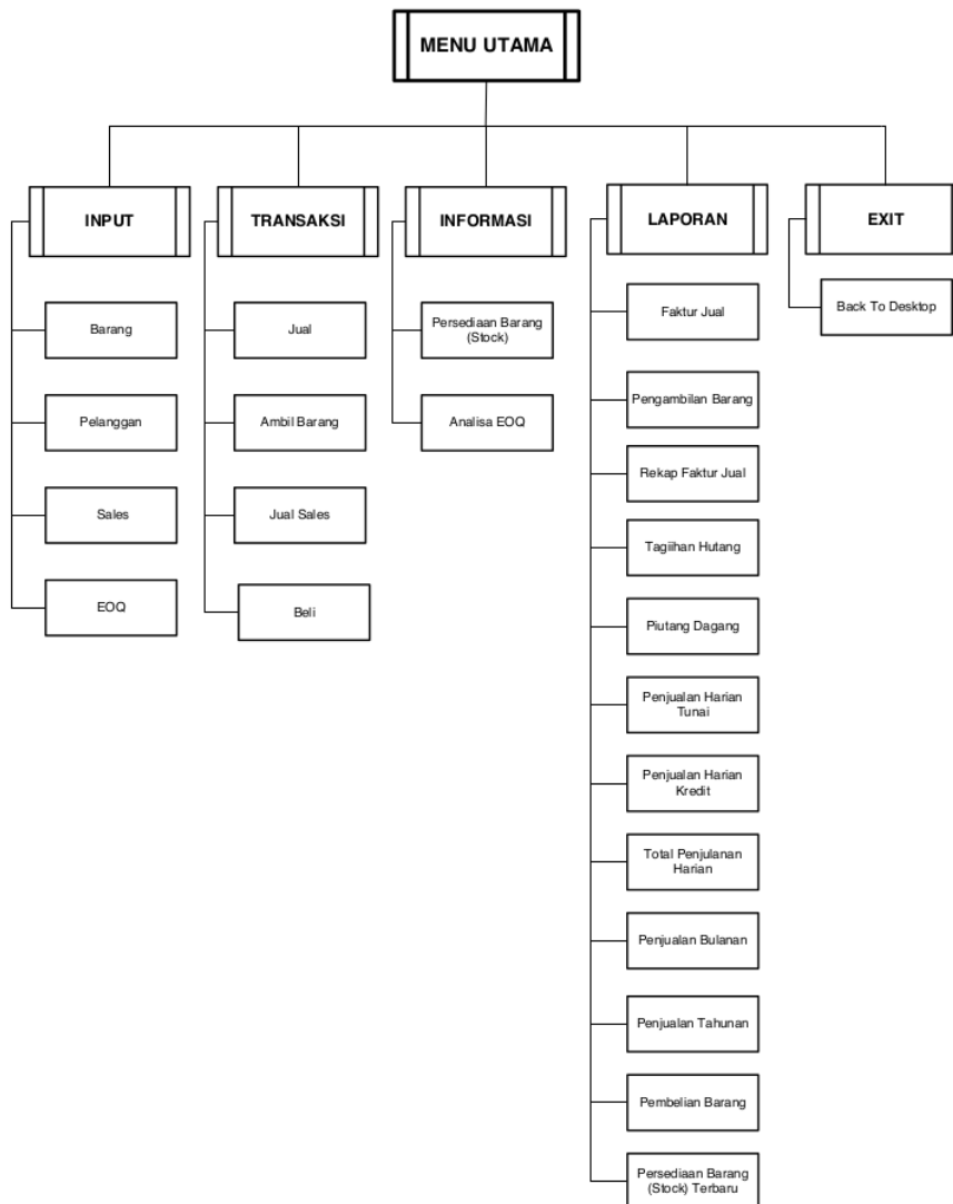
Gambar 6.6. Struktur Program
