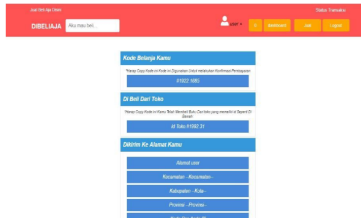
Gambar6.17 AntarmukaMenuCheckout
