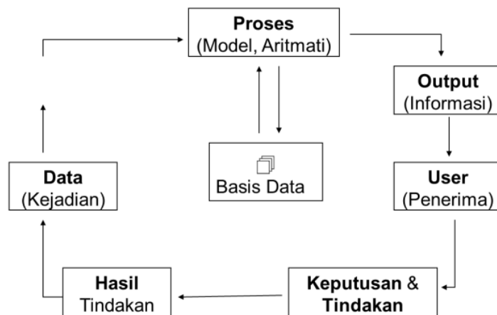
Gambar 1.2. Siklus Informasi
