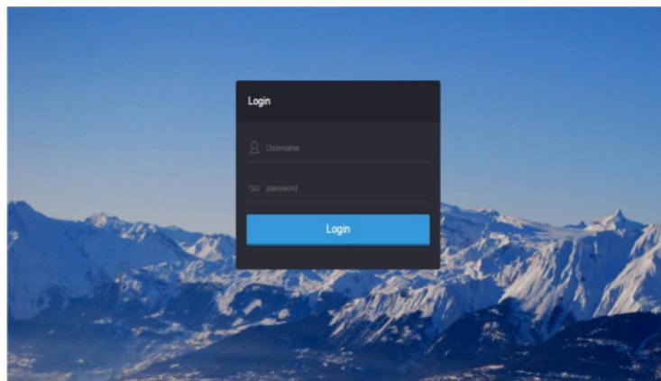
Gambar6.8 Antarmuka HalamanLoginAdmin
