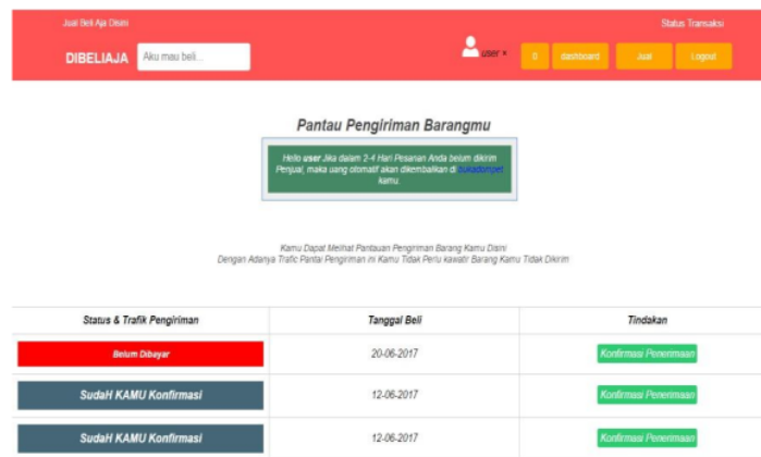
Gambar6.19 AntarmukaMenuStatus Transaksi
