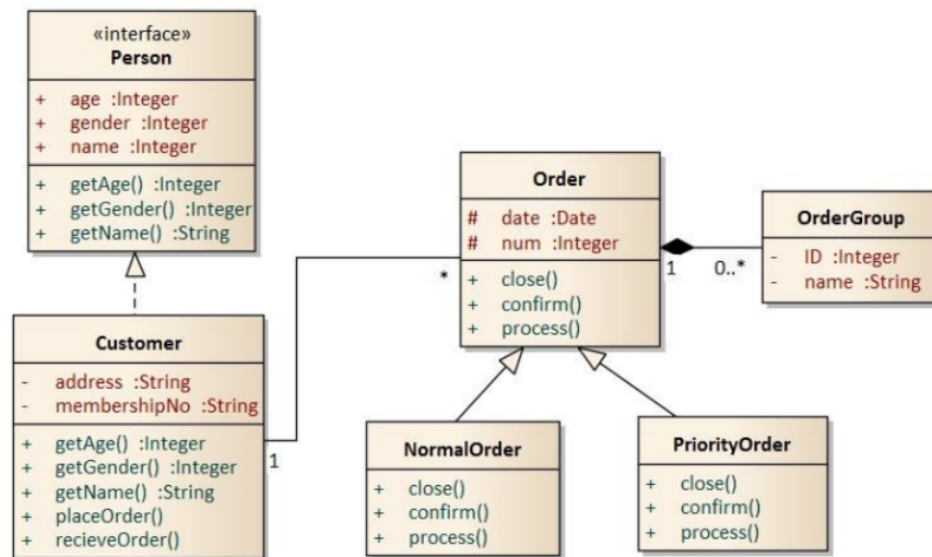
Gambar3.10.ClassDiagram
