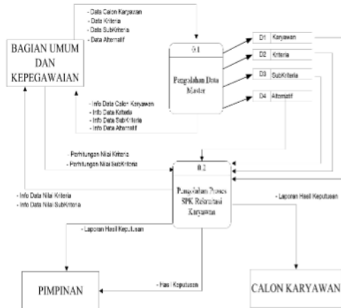
Gambar 5. DFD Level 0 SPK Penerimaan Karyawan
