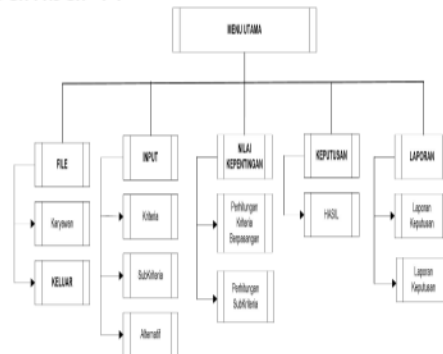
Gambar 7. Struktur Program
