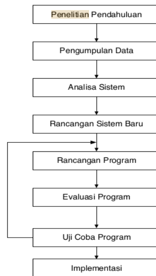
Gambar 3.1 Metodologi Penelitian
