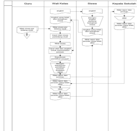
Gambar 1. Aliran Sistem Informasi (ASI) Baru
