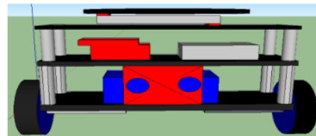
Gambar 6. Rancang Fisik Robot Tampak Belakang
