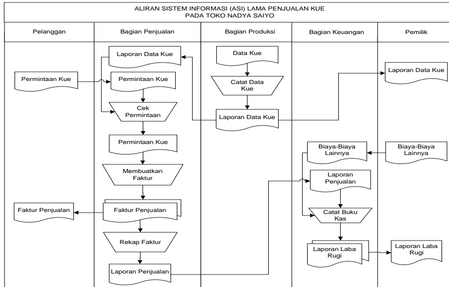
Gambar 3.1. Aliran Sistem Informasi Lama
