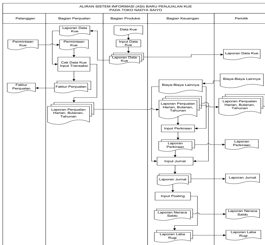
Gambar 3.2. Aliran Sistem Informasi Baru
